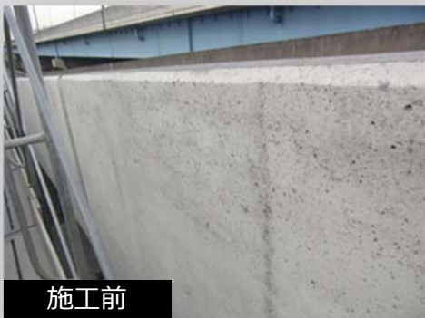
高架橋 剥落防止工事 324㎡ (東京都)
